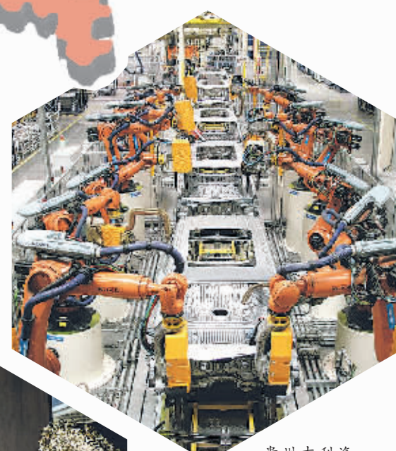
贵州吉利汽车制造有限公司生产线。(吉利汽车供图)
